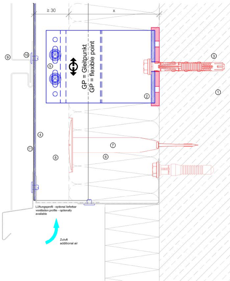
Vertikalschnitt - Sockelabschluss vertical section - base detail
